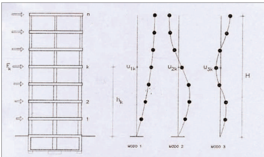
Modos de vibración en modelos planos de estructuras de pisos
